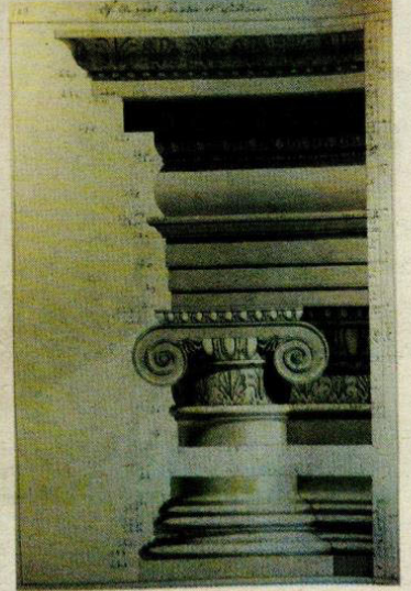
Laodikeia tiyatrosu, sahne önündeki yarım sütun düzeninin kaidesi, sütun başlığı ve saçaklık çizimi. (Çizim: Niholas Ravett, Env. 2013, 5005.2.38, © British Museum'un izniyle)
